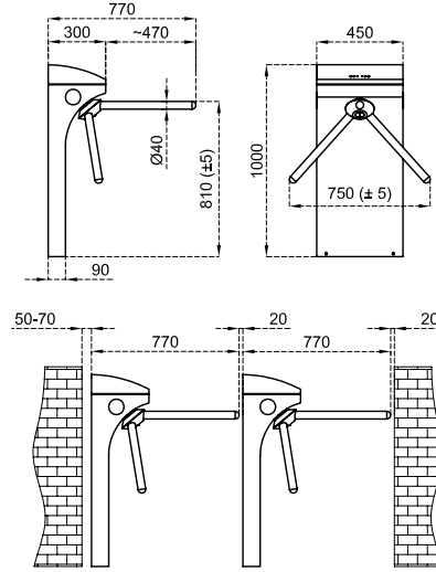
Ölçüler (mm)
