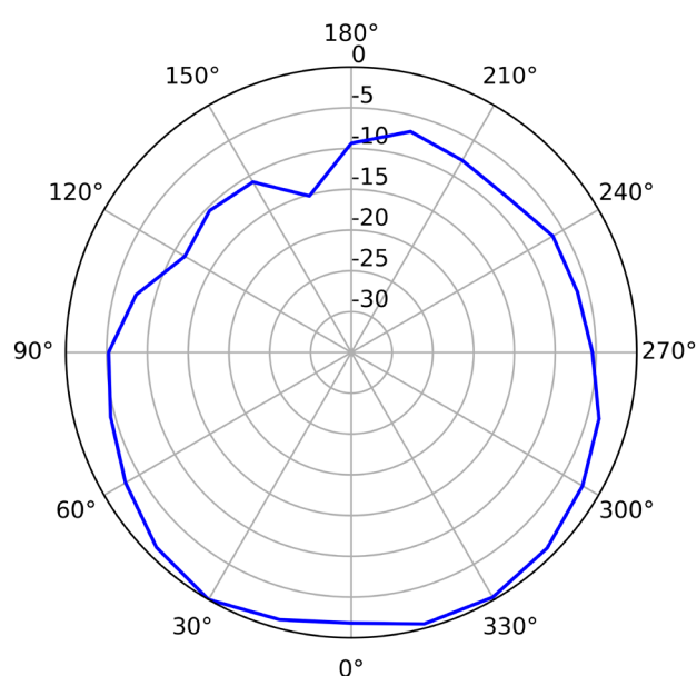
2.4GHz (Vertical)
