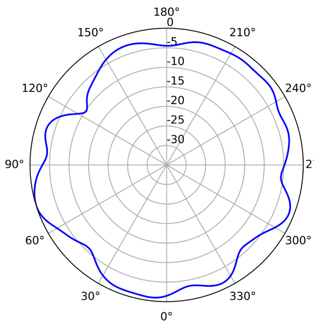
5GHz (Horizontal)
