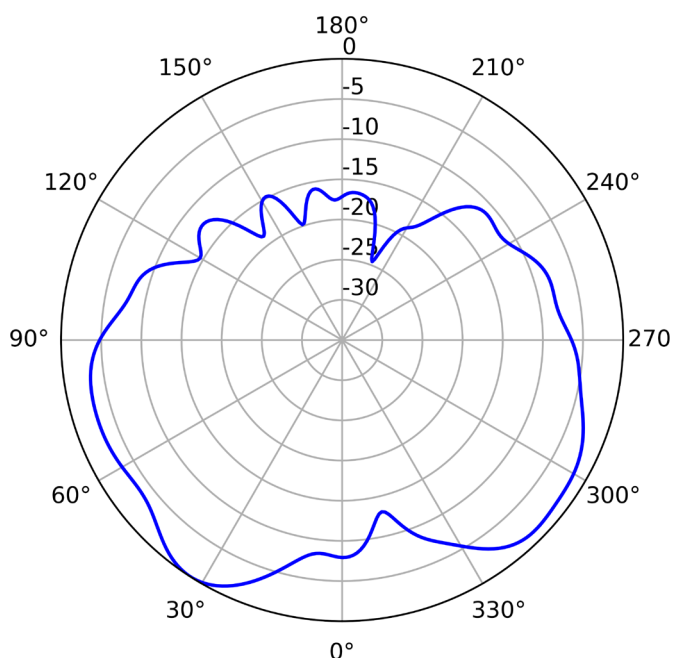
5GHz (Vertical)
