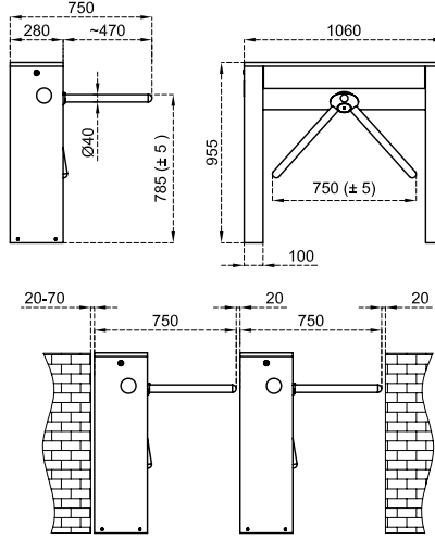
Ölçüler (mm)
