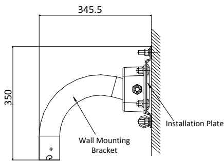
DS-1690ZJ-X Dimensions
